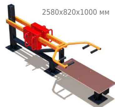
Премиум тренажер Жим лёжа с изменяемой нагрузкой
